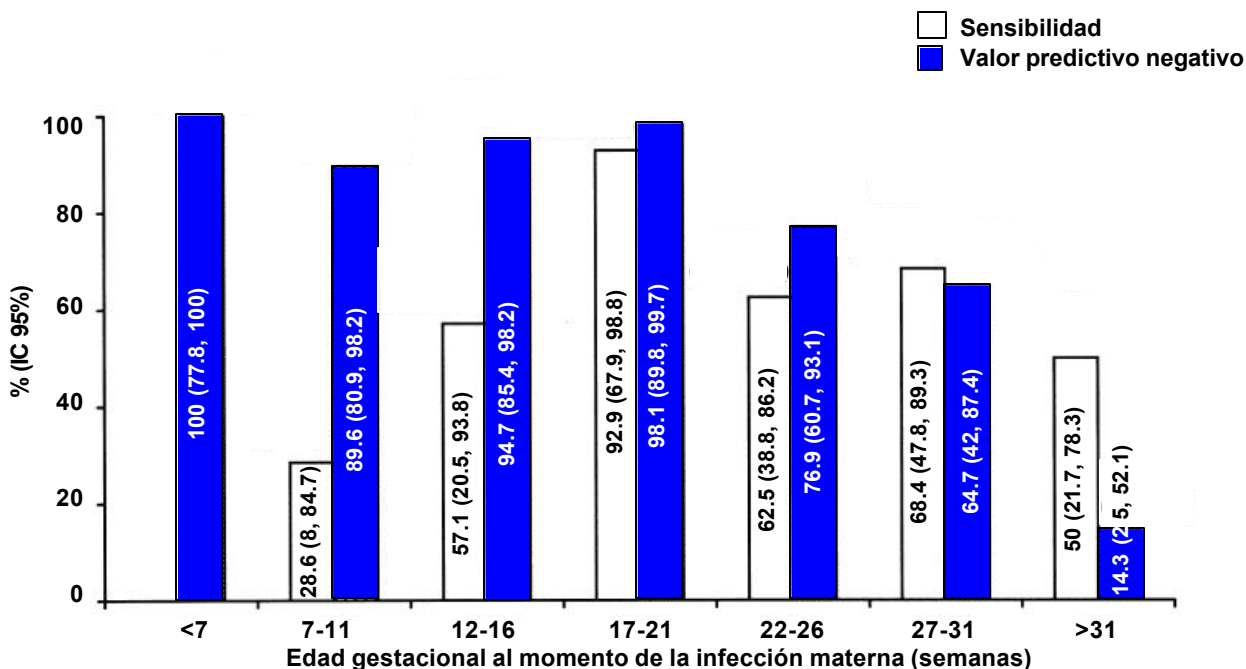
Gráfica 4. Diagnóstico prenatal de la toxoplasmosis congénita utilizando reacción en cadena de la polimerasa (PCR) en líquido amniótico, según la edad gestacional al momento de la infección materna (semanas). Adaptado de Romand et al. 54
