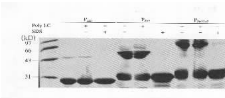
图 5 CaPKR-like Z\alpha 多肽的体外二聚化
