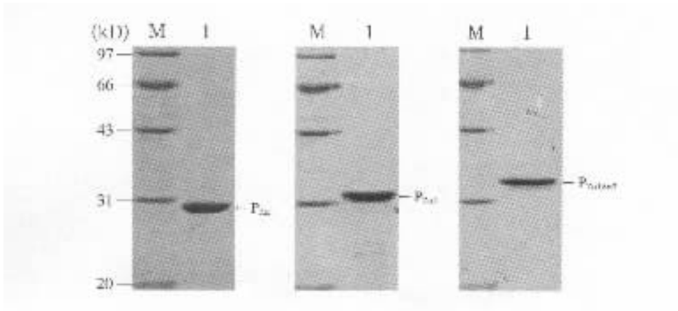
图 2 CaPKR-like Z\alpha 融合蛋白的亲和层析纯化
