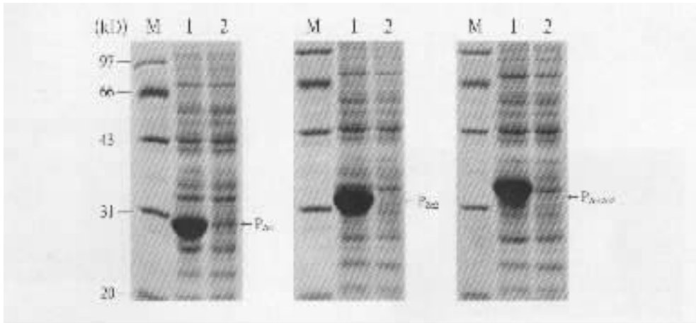
图 1 CaPKR-like 基因 Z\alpha 结构域的原核表达
