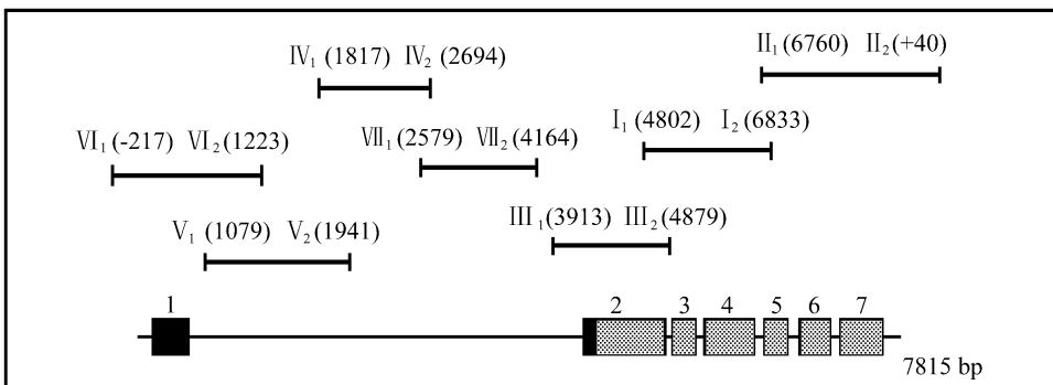
图 1 ebony 基因结构 (GenBank accession no. AJ224446) 引物所在位置及其扩增的片段
