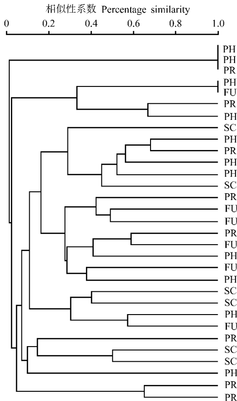
图 4 基于 Bray-Curtis 相似性系数，采用组间联法，以地表甲虫群落为属性对不同功能群的聚类分析图
