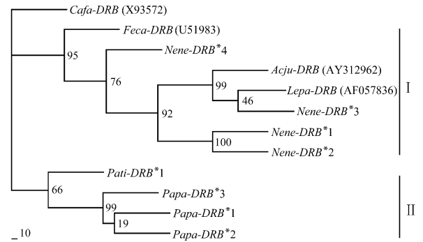
图 4 基于 MHC DRB 基因第二外元序列构建的 MP 树, 各分支上数字为 Bootstrap 1 000 次循环的自举检验值
