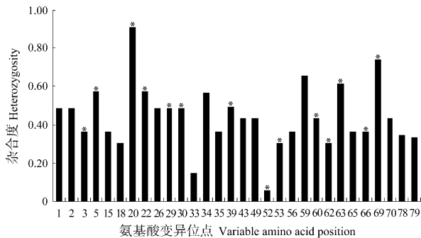
图 1 8 种氨基酸序列变异位点的平均杂合度
