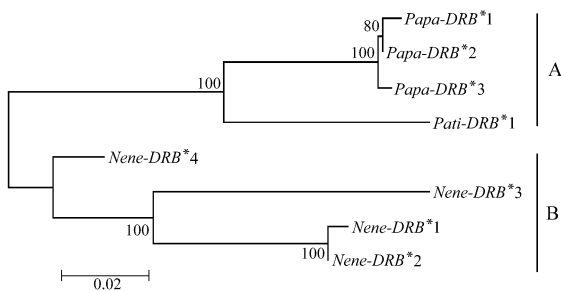
图 2 基于 8 种序列构建的 NJ 树, 各分支上数字为 Bootstrap 1 000 次循环的自举检验值
