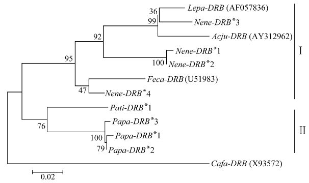
图 3 基于 MHC DRB 基因第二外元序列构建的 NJ 树, 各分支上数字为 Bootstrap 1 000 次循环的自举检验值
